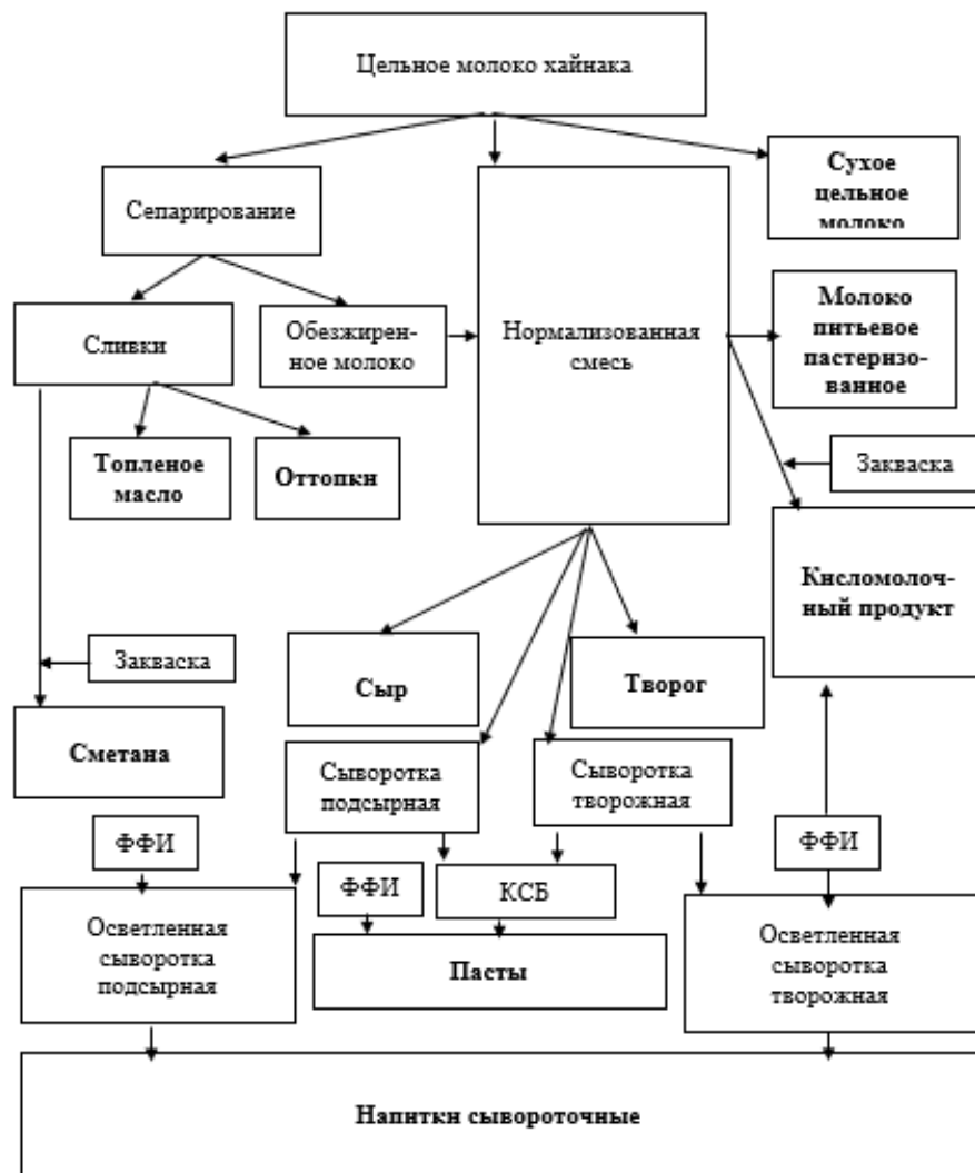
Рисунок 5.1 – Схема предлагаемой безотходной технологии переработки молока хайнака
