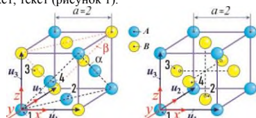
Рисунок 1 – Ячейки сверхструктуры L1_1 (слева) и L1_2 (справа)
