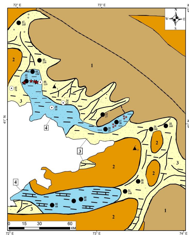
Рисунок 4.1 - Литолого-палеогеографическая карта среднеюрской эпохи (келловей). Масштаб 1:1500000. (На основе карты В.И. Троицкого [287], с нашими дополнениями).
