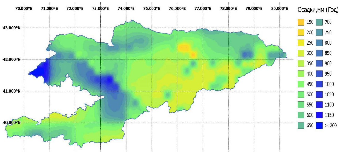
Рис. 4. Карта годовых сумм осадков за период январь 1998 – февраль 2014 гг. после приведения исходных спутниковых данных к показаниям метеостанций, полученная по спутниковым данным по разработанной технологии
