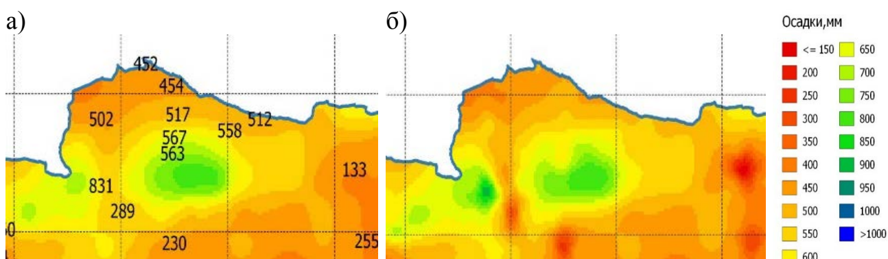
Рис. 1. Фрагмент карты годовых сумм осадков по модели ТМРА для части территории ССЗК без применения метода объективной интерполяции (а) и с его применением (б). Числа на а) соответствуют значения осадков (мм) по данным расположенных здесь метеостанций
